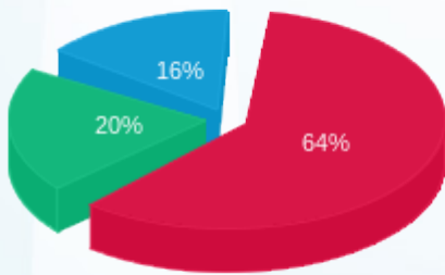
■ פסגה (Kwh 15,600.20) ■ גבע (Kwh 4,965.95) ■ שפל (Kwh 3,806.50)
