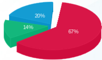
■ פסגה (Kwh 76,172.39) ■ גבע (Kwh 15,876.72) ■ שפל (Kwh 22,389.35)
