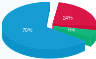
■ פסגה (10,837.25 Kwh) ■ גבע (2,392.25 Kwh) ■ שפל (31,586.40 Kwh)
