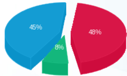
■ פסגה (NWh 37,080.49) 48% ■ גבע (NWh 6,030.98) 8% ■ שפל (NWh 34,942.03) 45%
