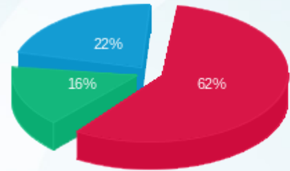
פסגה (Kwh 50,198.36) גבע (Kwh 12,881.25) שפל (Kwh 18,096.43)
