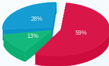
■ פסגה (31,852.87 Kwh) ■ גבע (7,081.48 Kwh) ■ שפל (14,967.42 Kwh)
