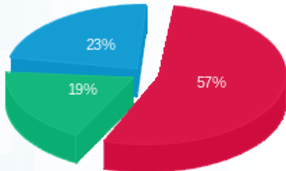
■ פסגה (Kwh 115,159.60) ■ גבע (Kwh 38,299.80) ■ שפל (Kwh 46,932.40)
