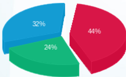
■ פסגה (45,389.61 Kwh) ■ גבע (24,524.85 Kwh) ■ שפל (33,648.22 Kwh)
