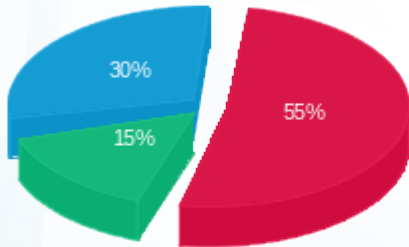
■ פסגה (116,161.51 Kwh) ■ גבע (32,939.95 Kwh) ■ שפל (63,942.94 Kwh)
