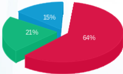
■ פסגה (199,971.04 Kwh) ■ גבע (66,380.99 Kwh) ■ שפל (45,847.94 Kwh)
