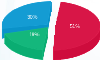
■ פסגה (96,096.77 Kwh) ■ גבע (35,636.73 Kwh) ■ שפל (55,882.83 Kwh)
