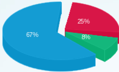
■ פסגה (Kwh 730,264.68) ■ גבע (Kwh 242,293.93) ■ שפל (Kwh 1,954,441.72)
