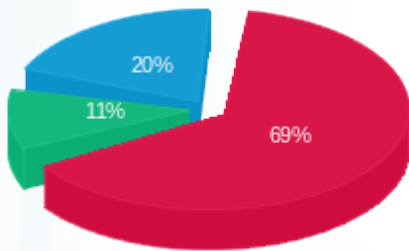
■ פסגה (37,515.10 Kwh) ■ גבע (5,796.30 Kwh) ■ שפל (11,117.35 Kwh)
