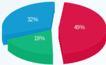
פסגה (Kwh 445,969.29) גבע (Kwh 172,741.58) שפל (Kwh 297,662.64)
