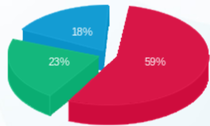
■ פסגה (Kwh 150,610.73) ■ גבע (Kwh 57,517.12) ■ שפל (Kwh 46,889.85)
