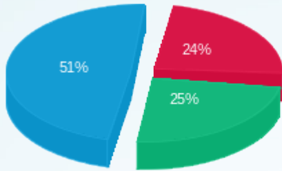
פסגה (Kwh 17,095.26) ■ גבע (Kwh 17,856.73) ■ שפל (Kwh 36,170.46) ■
