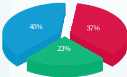
■ פסגה (122,733.27 Kwh) ■ גבע (77,252.09 Kwh) ■ שפל (134,643.55 Kwh)
