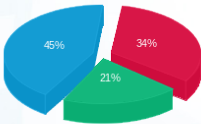
■ פסגה (Kwh 33,775.84) ■ גבע (Kwh 20,820.99) ■ שפל (Kwh 44,042.82)
