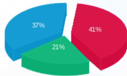
■ פסגה (Kwh 15,861.13) ■ גבע (Kwh 8,145.17) ■ שפל (Kwh 14,322.73)
