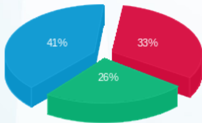
■ פסגה (Kwh 338,622.73) ■ גבע (Kwh 262,882.54) ■ שפל (Kwh 418,775.44)
