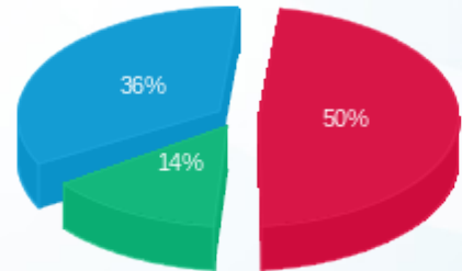
■ פסגה (Kwh 23,544.97) ■ גבע (Kwh 6,626.48) ■ שפל (Kwh 16,648.96)
