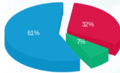
■ פסגה (Kwh 82,264.65) ■ גבע (Kwh 17,696.25) ■ שפל (Kwh 156,327.15)
