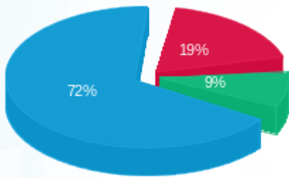
■ פסגה (20,775.30 Kwh) ■ גבע (9,899.50 Kwh) ■ שפל (78,437.00 Kwh)
