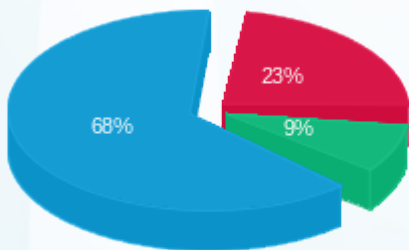
■ פסגה (23,037.00 Kwh) ■ גבע (8,509.25 Kwh) ■ שפל (67,848.35 Kwh)
