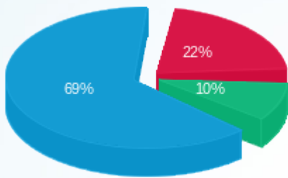
■ פסגה (Kwh 18,958.52) ■ גבע (Kwh 8,435.16) ■ שפל (Kwh 59,747.81)
