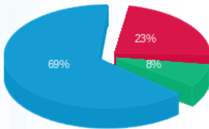
■ פסגה (110,473.04 Kwh) ■ גבע (36,705.38 Kwh) ■ שפל (326,584.33 Kwh)
