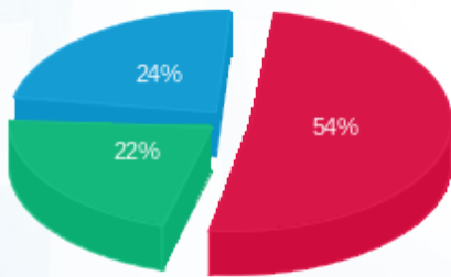
■ פסגה (Kwh 434,543.29) ■ גבע (Kwh 181,377.20) ■ שפל (Kwh 193,191.71)
