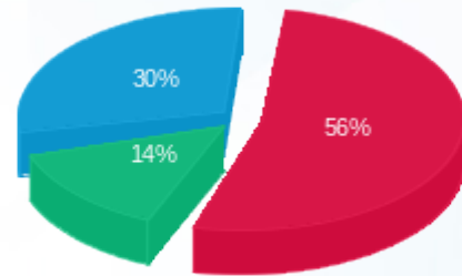
■ פסגה (Kwh 39,712.85) ■ גבע (Kwh 10,129.46) ■ שפל (Kwh 21,327.31)
