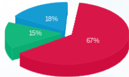
■ פסגה (Kwh 11,751.89) ■ גבע (Kwh 2,630.94) ■ שפל (Kwh 3,062.03)
