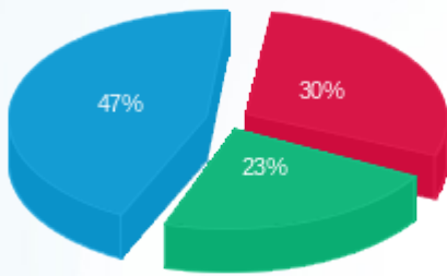
■ פסגה (Kwh 67,762.30) ■ גבע (Kwh 52,539.90) ■ שפל (Kwh 104,869.60)
