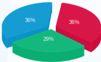
■ פסגה (12,656.00 Kwh) ■ גבע (10,173.55 Kwh) ■ שפל (12,777.65 Kwh)
