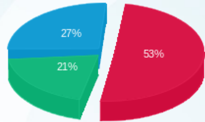
פסגה (₪ 36,164.06) גבע (₪ 14,009.48) שפל (₪ 18,129.01)
