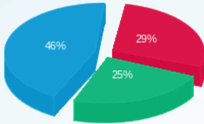
פסגה (Kwh 33,719.40) גבע (Kwh 28,737.40) שפל (Kwh 53,859.20)
