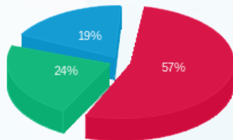
■ פסגה (Kwh 17,219.20) 57% ■ גבע (Kwh 7,091.20) 24% ■ שפל (Kwh 5,664.80) 19%
