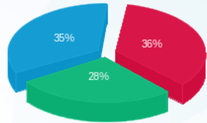
■ פסגה (Kwh 258,235.85) ■ גבע (Kwh 202,086.15) ■ שפל (Kwh 249,766.60)
