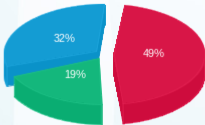
■ פסגה (Kwh 25,092.26) ■ גבע (Kwh 9,883.92) ■ שפל (Kwh 16,485.77)
