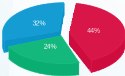
■ פסגה (Kwh 84,879.70) ■ גבע (Kwh 47,033.10) ■ שפל (Kwh 62,305.60)
