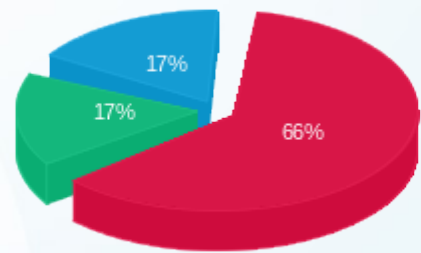
■ פסגה (Kwh 197,936.88) ■ גבע (Kwh 49,492.89) ■ שפל (Kwh 52,149.95)
