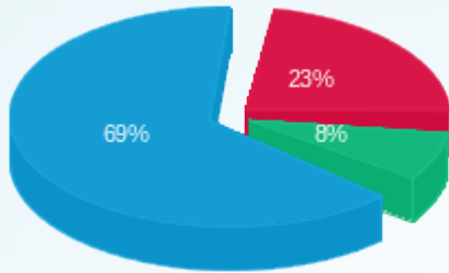
פסגה (Kwh 467,987.90) ■ גבע (Kwh 157,653.06) ■ שפל (Kwh 1,398,630.14) ■
