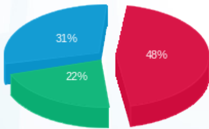
■ פסגה (Kwh 286,744.94) ■ גבע (Kwh 129,267.74) ■ שפל (Kwh 182,745.65)
