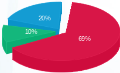
פסגה (Kwh 22,065.71) ■ גבע (Kwh 3,335.15) ■ שפל (Kwh 6,426.12) ■
