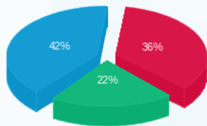
פסגה (Kwh 82,186.79) 42% גבע (Kwh 49,049.60) 22% שפל (Kwh 94,162.43) 36%
