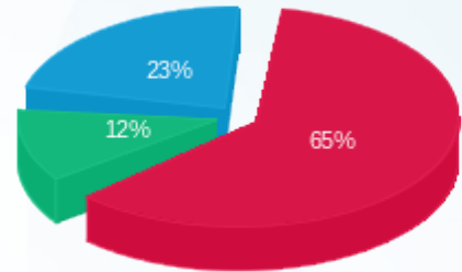
■ פסגה (Kwh 26,706.46) ■ גבע (Kwh 4,803.23) ■ שפל (Kwh 9,352.79)
