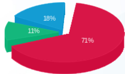
■ פסגה (Kwh 27,855.86) ■ גבע (Kwh 4,371.06) ■ שפל (Kwh 6,911.41)
