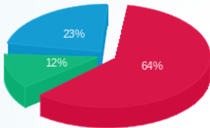
■ פסגה (Kwh 61,302.52) ■ גבע (Kwh 11,609.72) ■ שפל (Kwh 22,244.64)
