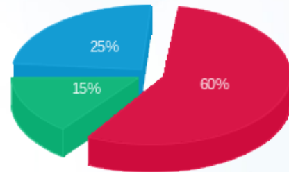
■ פסגה (73,522.35 Kwh) ■ גבע (18,218.95 Kwh) ■ שפל (30,439.10 Kwh)
