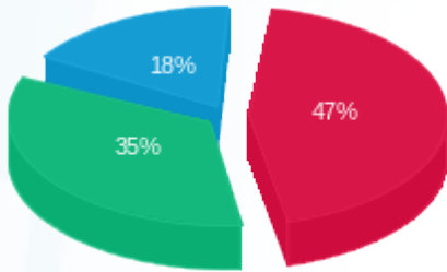
פסגה (Kwh 45,635.42) ■ גבע (Kwh 34,195.20) ■ שפל (Kwh 17,124.68) ■
