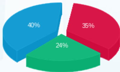
■ פסגה (Kwh 142,589.45) ■ גבע (Kwh 97,806.28) ■ שפל (Kwh 163,427.00)
