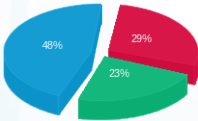
■ פסגה (99,876.99 Kwh) ■ גבע (79,766.27 Kwh) ■ שפל (163,017.28 Kwh)
