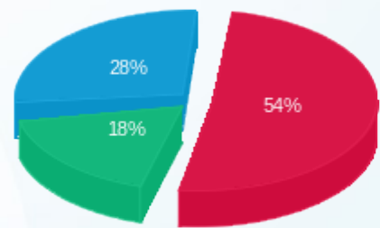
■ פסגה (3,628.63 Kwh) 28% ■ גבע (1,226.32 Kwh) 18% ■ שפל (1,904.16 Kwh) 54%
