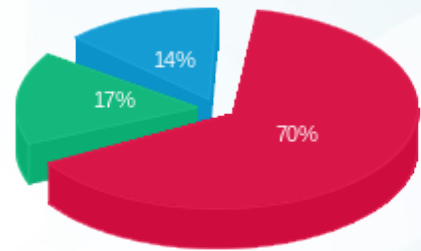
■ פסגה (32,156.97 Kwh) ■ גבע (7,632.23 Kwh) ■ שפל (6,426.03 Kwh)
