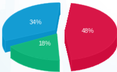
■ פסגה (126,892.40 Kwh) ■ גבע (47,299.10 Kwh) ■ שפל (88,313.30 Kwh)
