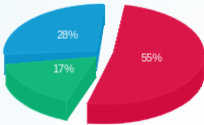
פסגה (173,045.79 Kwh) ■ גבע (54,595.75 Kwh) ■ שפל (88,159.74 Kwh) ■
